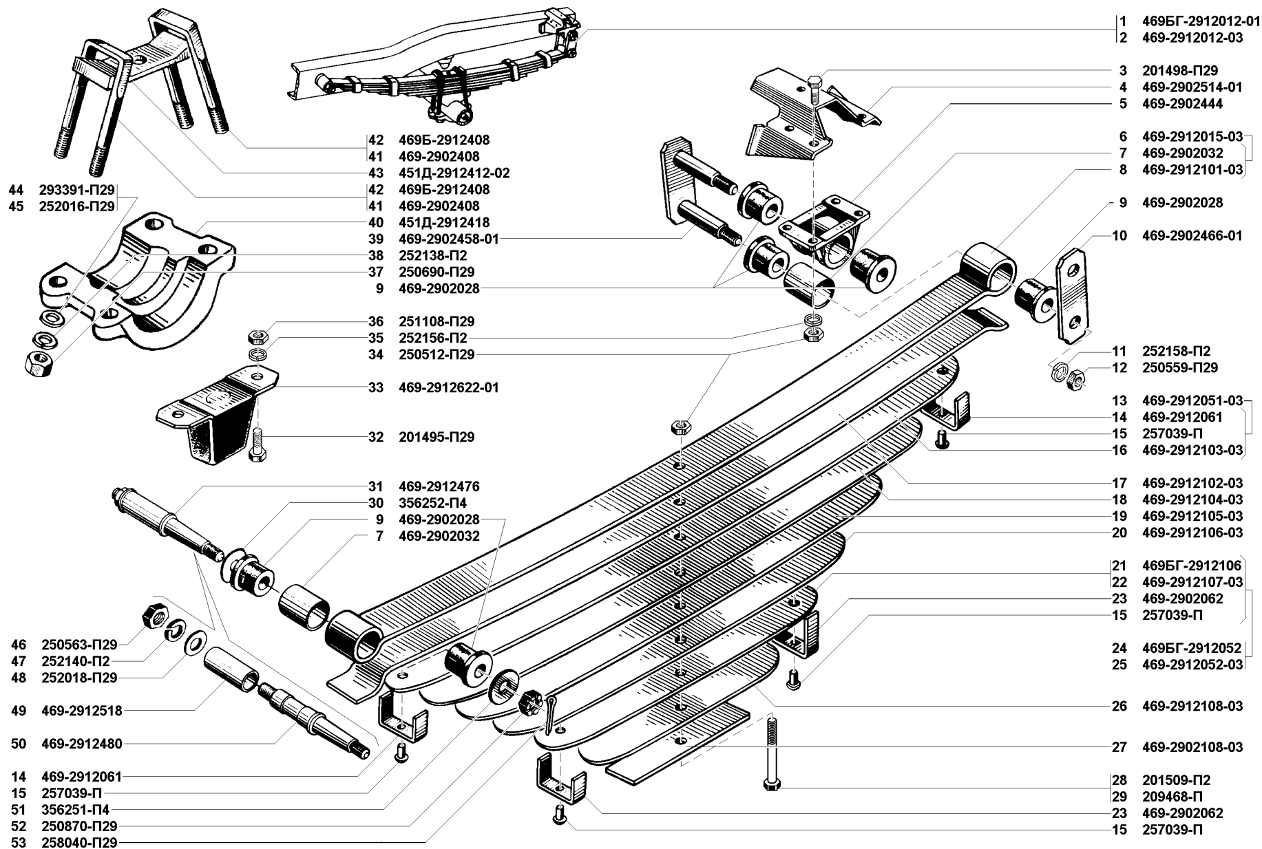
Рис. 88. Рессоры задние (2912)
