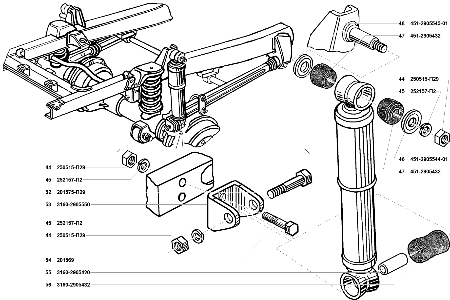
Рис. 87. Амортизаторы передние (2905)/3
